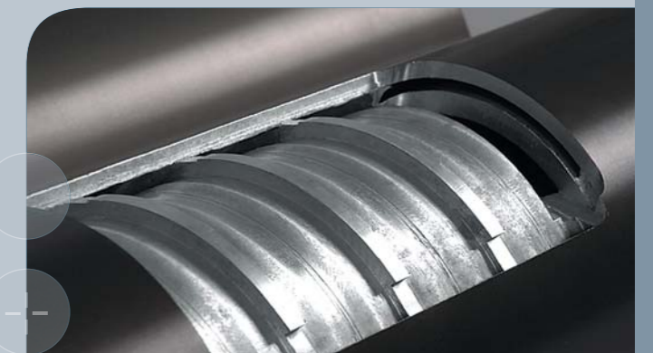
Querschnitt: Kühlwalze mit Innenspirale z. B. Kühlwalzen für UV-Trockner, Etikettendruck.
